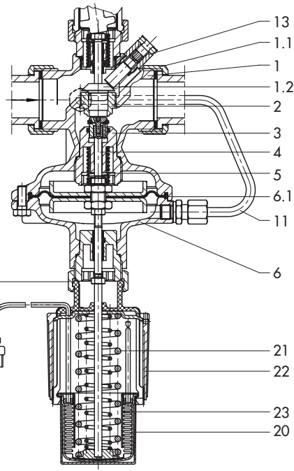
Type 2489/5827, PN 25 - Exécution avec corps taraudé -
