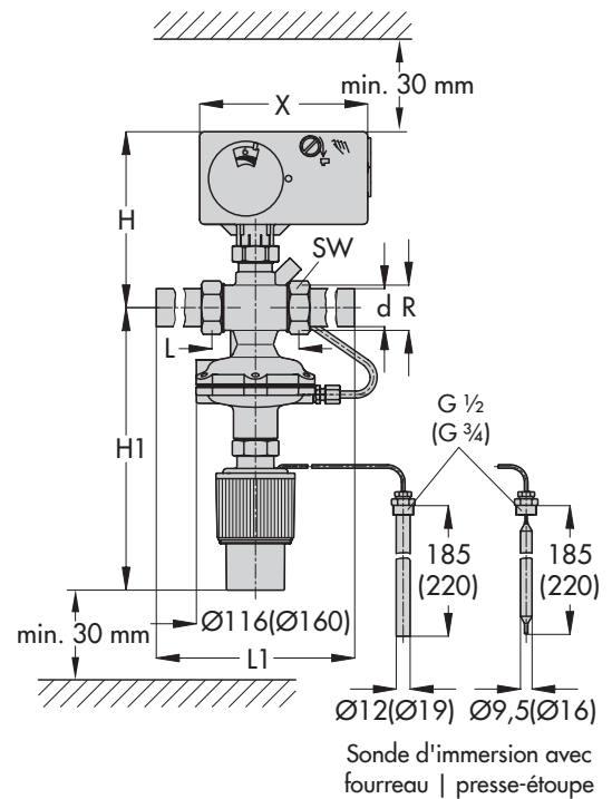
Type 2489/5827 ou 5724 (5725) Raccords vissés avec embouts à souder
