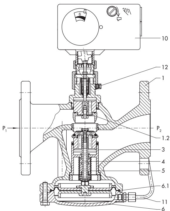
Type 2488/5827, PN 25, DN 32 à 50 - Exécution avec corps à brides -
