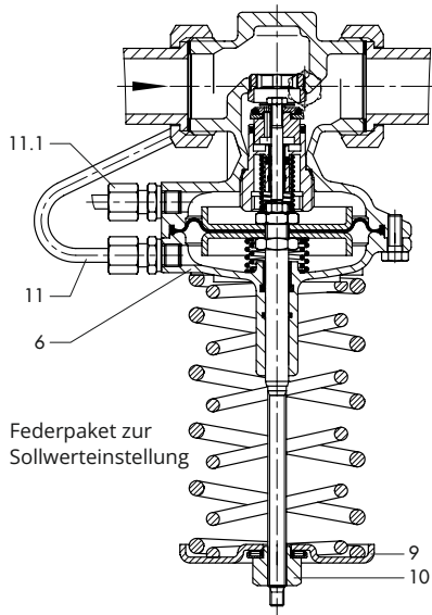
Typ 45-2 · Standardausführung (0,5 bis 2 bar/1 bis 4 bar/6 bis 10,5 bar)
