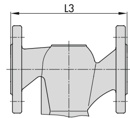
Flanschgehäuse DN 32, 40 und 50
