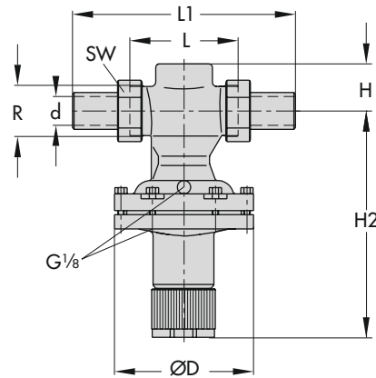
Typ 45-2 und 45-4 1) , DN 15 bis 32: 0,1 bis 0,5 bar und 0,1 bis 1 bar und 2,4 bis 6,3 bar
