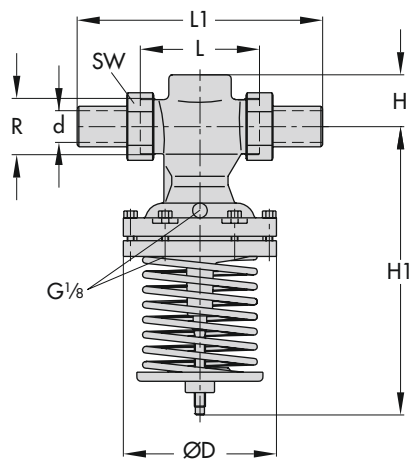
Typ 45-2 und 45-4 1) , DN 15 bis 32: 0,5 bis 2 bar und 1 bis 4 bar und 6 bis 10,5 bar DN 40/50, alle Sollwertbereiche
