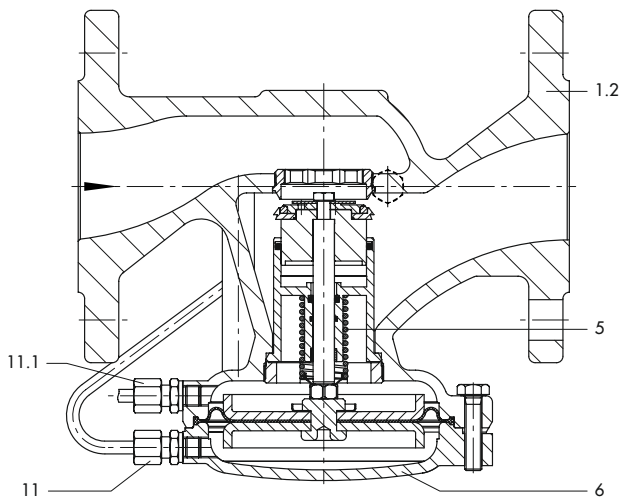
Typ 45-1 · Ausführung mit Flanschventil (DN 32, 40 und 50)
