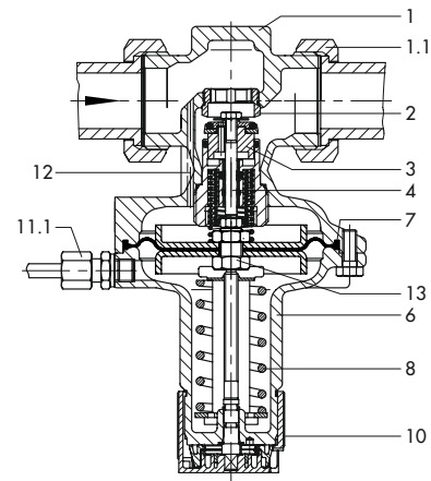
Regler für den Einbau in die Minusdruck-Leitung
