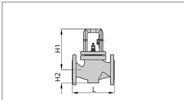
Afbeelding 13: Type 3241 · tot ontwerpdiameters DN 150/ NPS 6/DN 150A
