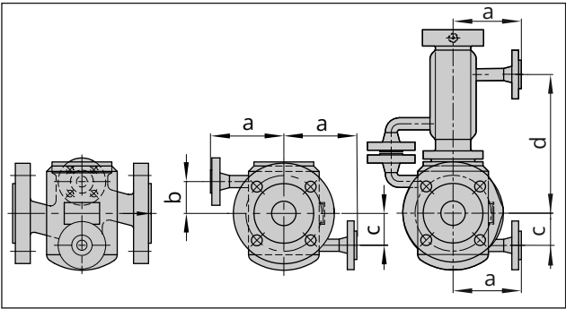
Afbeelding 12: Type 3241 met verwarmingsmantel vanaf ontwerpdiаметer DN 150/NPS 6 · in de afbeelding rechts met isoleer-/balgdeel
