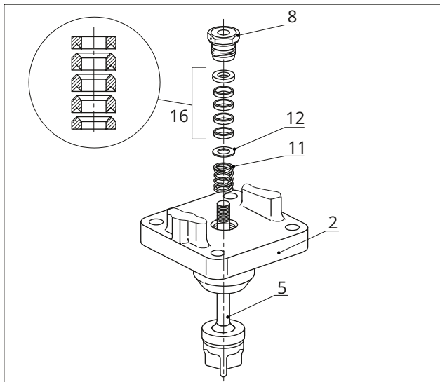
Afbeelding 26: Klepsteelpakking standaard
