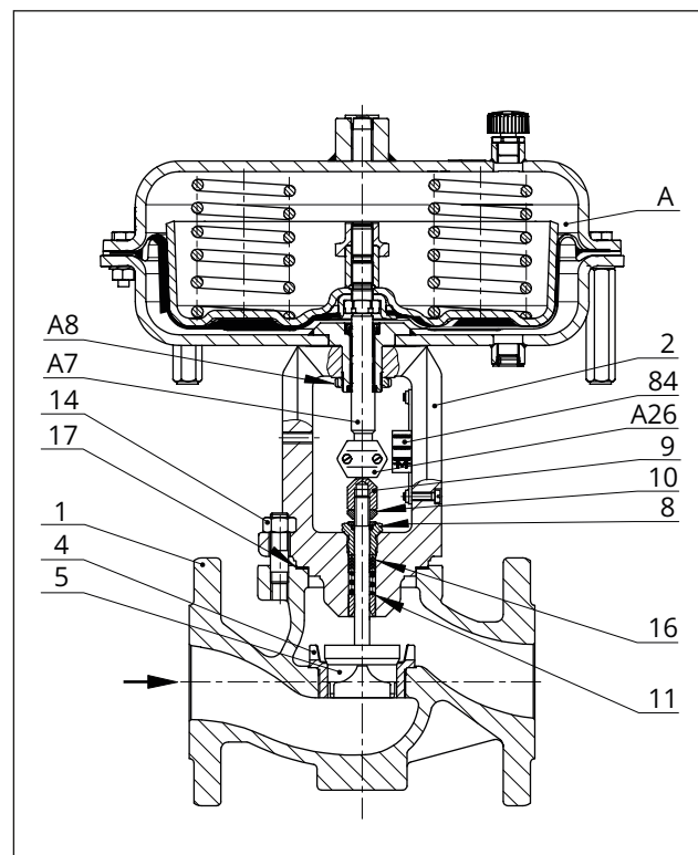
Afbeelding 24: Regelventiel van het type 3241-1 met pneumatische aandrijving van het type 3271, behuizing tot DN 150/NPS 6
