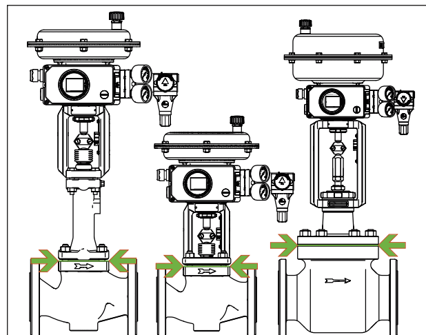
Afbeelding 15: Grenzen van de isolatie van regelventielen (voorbeeldweergave)
