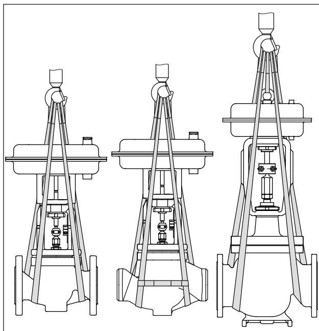
Afbeelding 14: Hijspunten aan het regelventiel: tot DN 150/NPS 6 met flenzen (links) en met laseinden (midden) · vanaf DN 150/NPS 6 met aanvullend draagoog aan de aandrijving (rechts)
