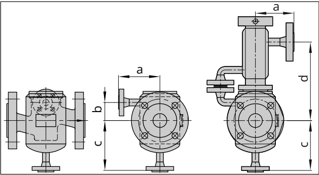
Afbeelding 11: Type 3241 met verwarmingsmantel tot ontwerpdiаметer DN 100/NPS 4 · in de afbeelding rechts met isoleer-/balgdeel
