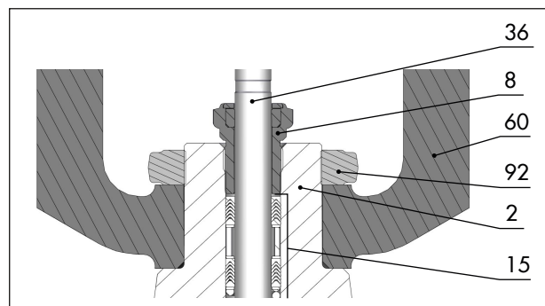
Afbeelding 22: Pakking met schroefdraadbus centraal aangebracht (voorbeeldweergave)
