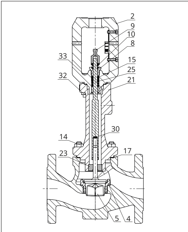
Afbeelding 25: Type 3241 in de uitvoering met isoleerdeel
