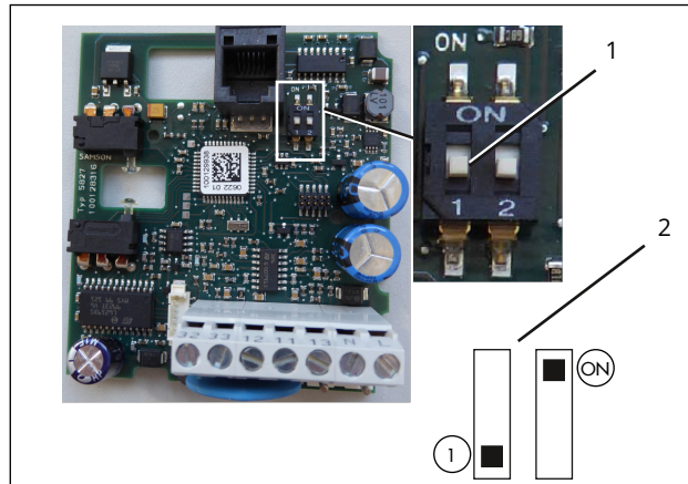
Bild 16: Funktionsschalter bei Ausführung 24 V
