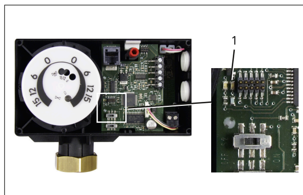
Bild 15: Position der LEDs bei Ausführung 85 bis 264 V
