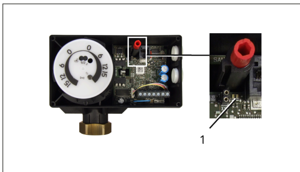
Bild 30: Position der LEDs bei Ausführung 24 V
