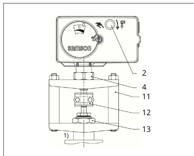
Bild 9: Formschlüssiger Anbau mit Kupplung, z. B. mit Joch an Ventil der Baureihe V2001
