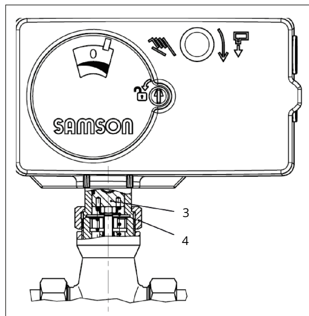
Bild 28: Kraftschlüssiger Anbau mit Überwurfmutter, z. B. an Ventil Typ 3222
