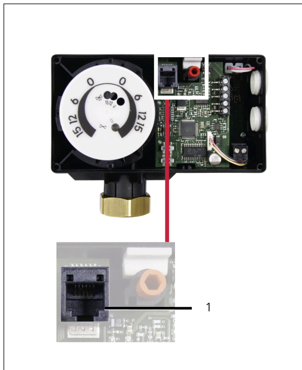
Bild 2: Serielle Schnittstelle
