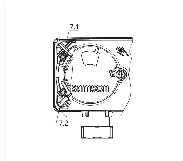
Bild 23: Einsteller für Grenzkontakte
