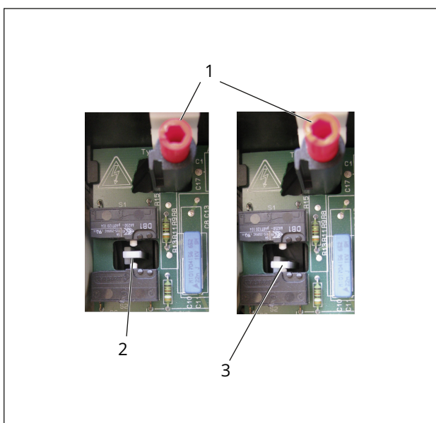
Bild 20: Stellachse und Endlagenschalter
