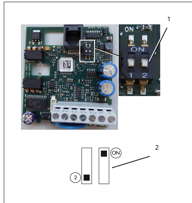
Bild 18: Wirkrichtungsschalter bei Ausführung 24 V
