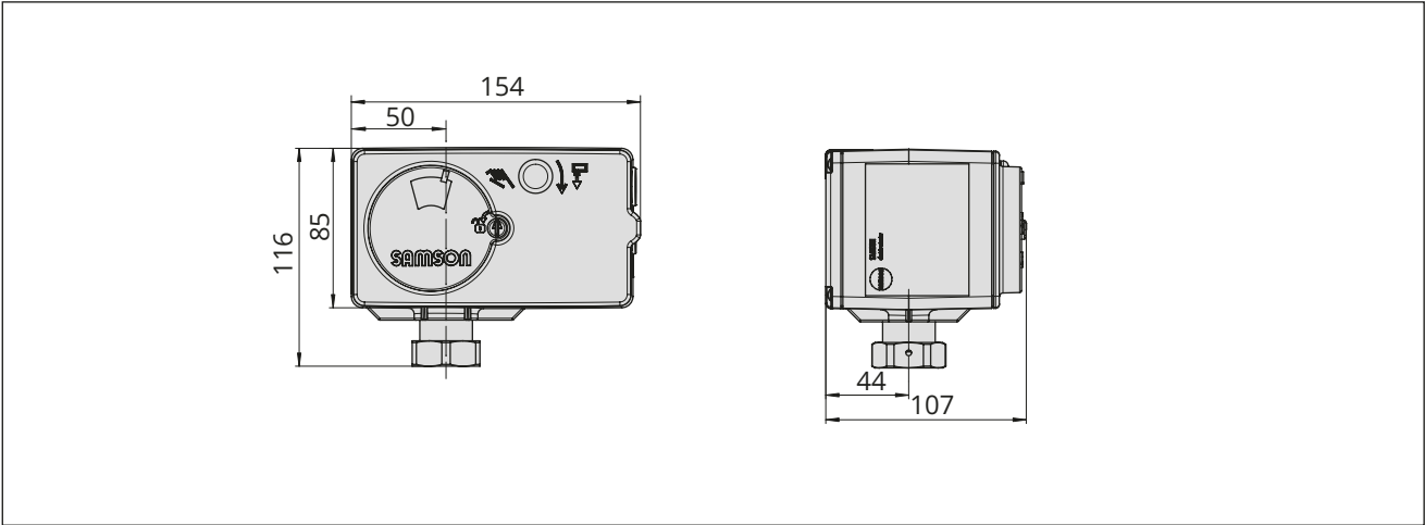
Bild 3: Maße in mm · kraftschlüssiger Anbau
