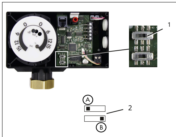
Bild 22: Funktionsschalter bei Ausführung 85 bis 264 V
