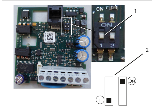
Bild 21: Funktionsschalter bei Ausführung 24 V
