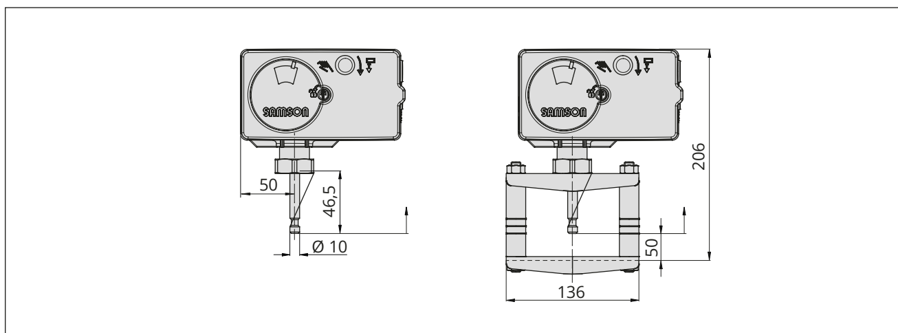
Bild 4: Maße in mm · formschlüssiger Anbau
