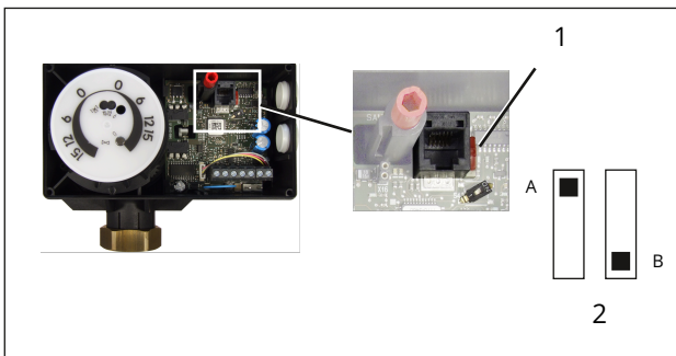
Bild 32: Wirkrichtungsschalter bei Ausführung 24 V
