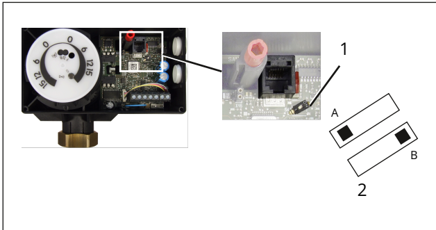
Bild 31: Funktionsschalter bei Ausführung 24 V
