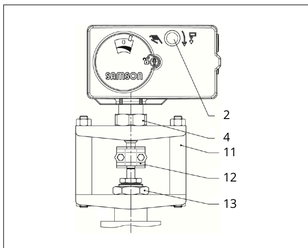
Bild 29: Formschlüssiger Anbau mit Kupplung, z. B. mit Joch an Ventil
