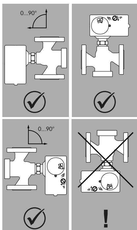
Bild 5: Einbaulage
