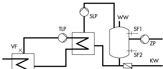
Bild 19: Aufbau eines Speicherladesystems
