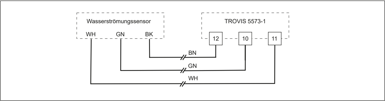
Bild 8: Wasserströmungssensor
