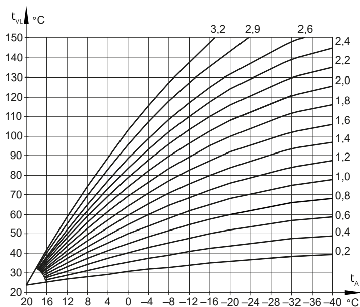
Bild 15: Steigungskennlinien
