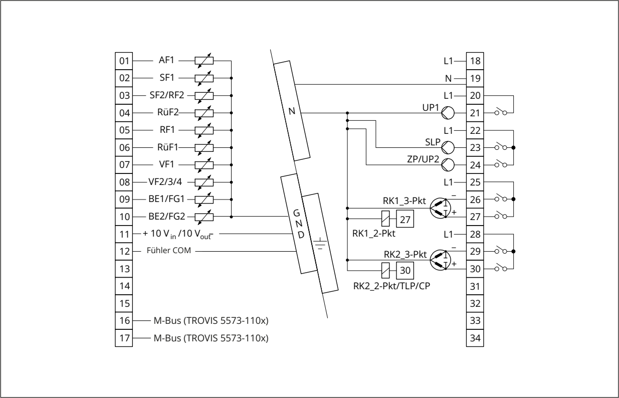
Bild 5: Elektrischer Anschluss des Reglers TROVIS 5573 mit hohem Geh user ckteil
