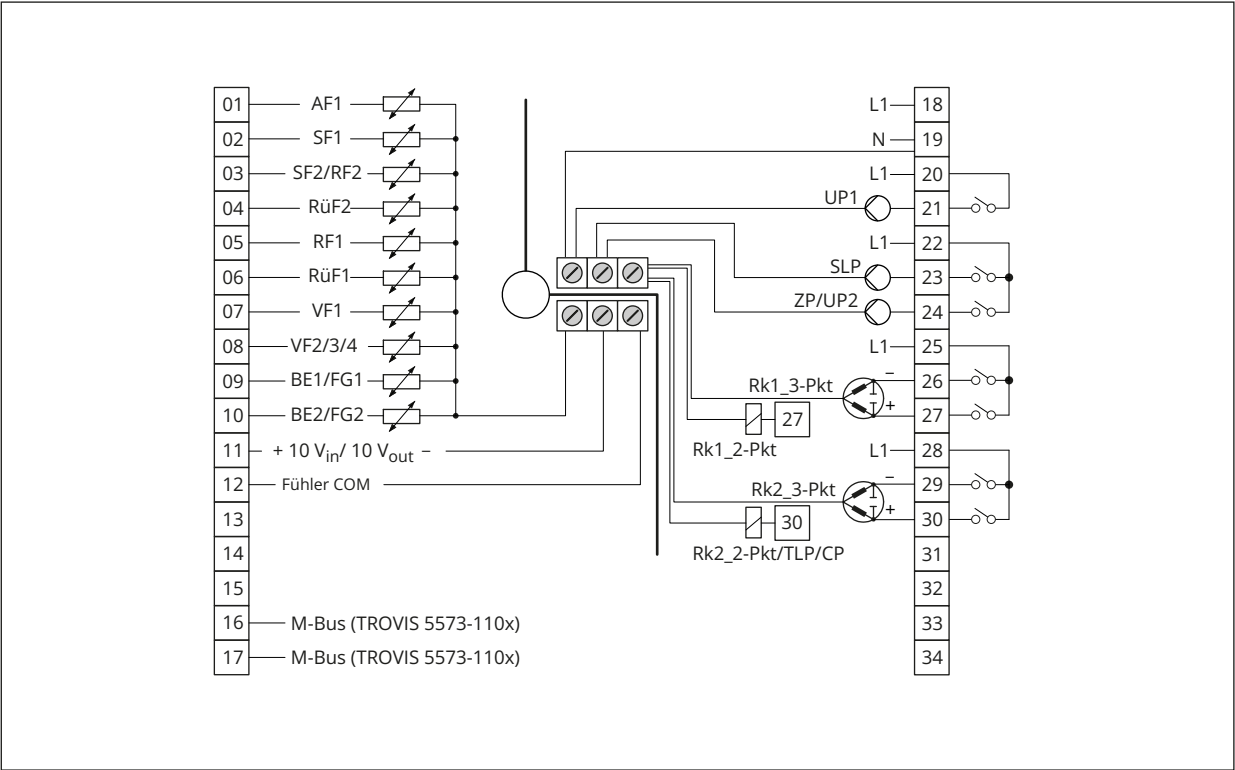
Bild 4: Elektrischer Anschluss des Reglers TROVIS 5573 mit Standard-Geh user ckteil
