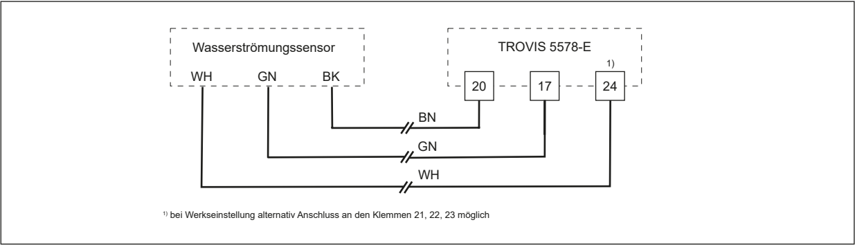
Bild 8: Wasserströmungssensor
